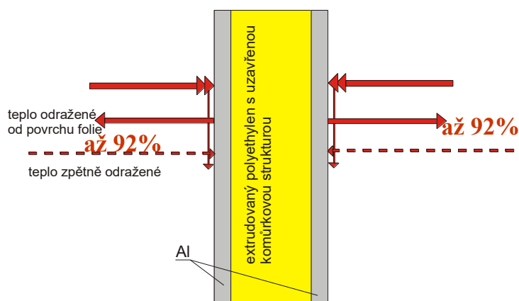
Obr. 2 Celkový tepelný tok
