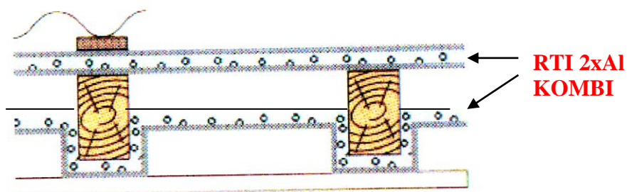
Obr. 4 Šikmá střešní konstrukce s ocelovým plechem
