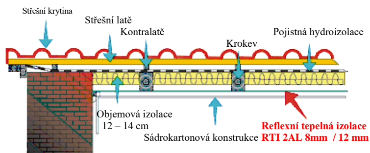
Obr. 3 Šikmá střešní konstrukce
